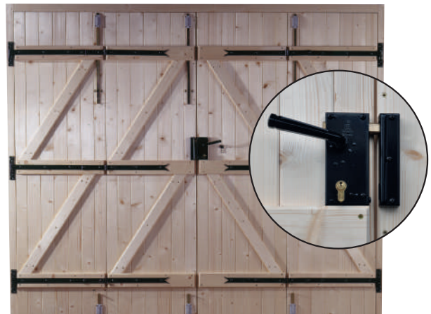
Porte de garage 4 vantaux repliables, serrure 1 point, verrou baïonnette, bâti 65 x 55 mm, avec bâti cintré dessous sans seuil - Sapin du Nord.
