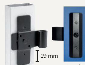
Équerre réglable EASY pour volets à cadre alu uniquement
